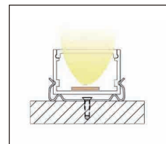
取付模式図
